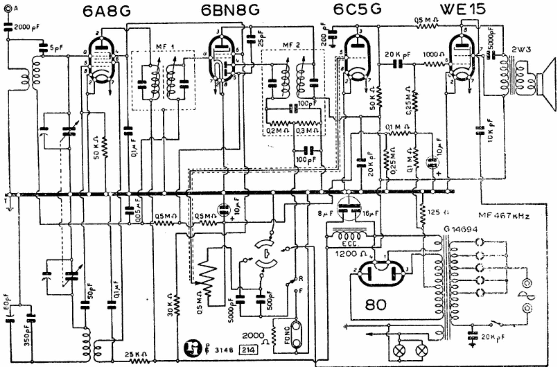
Lo schema elettrico del mod. 438 Siare
